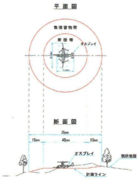
ヘリコプター着陸帯平面及び断面形状
